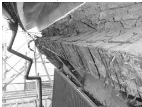
軒廻り装飾部の修理の様子 (ヤマニ邸)
