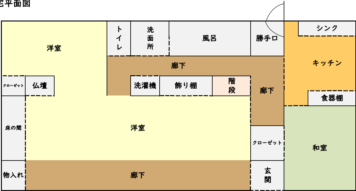
居宅平面図
