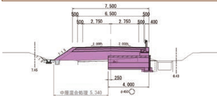
改良後 標準横断面図
